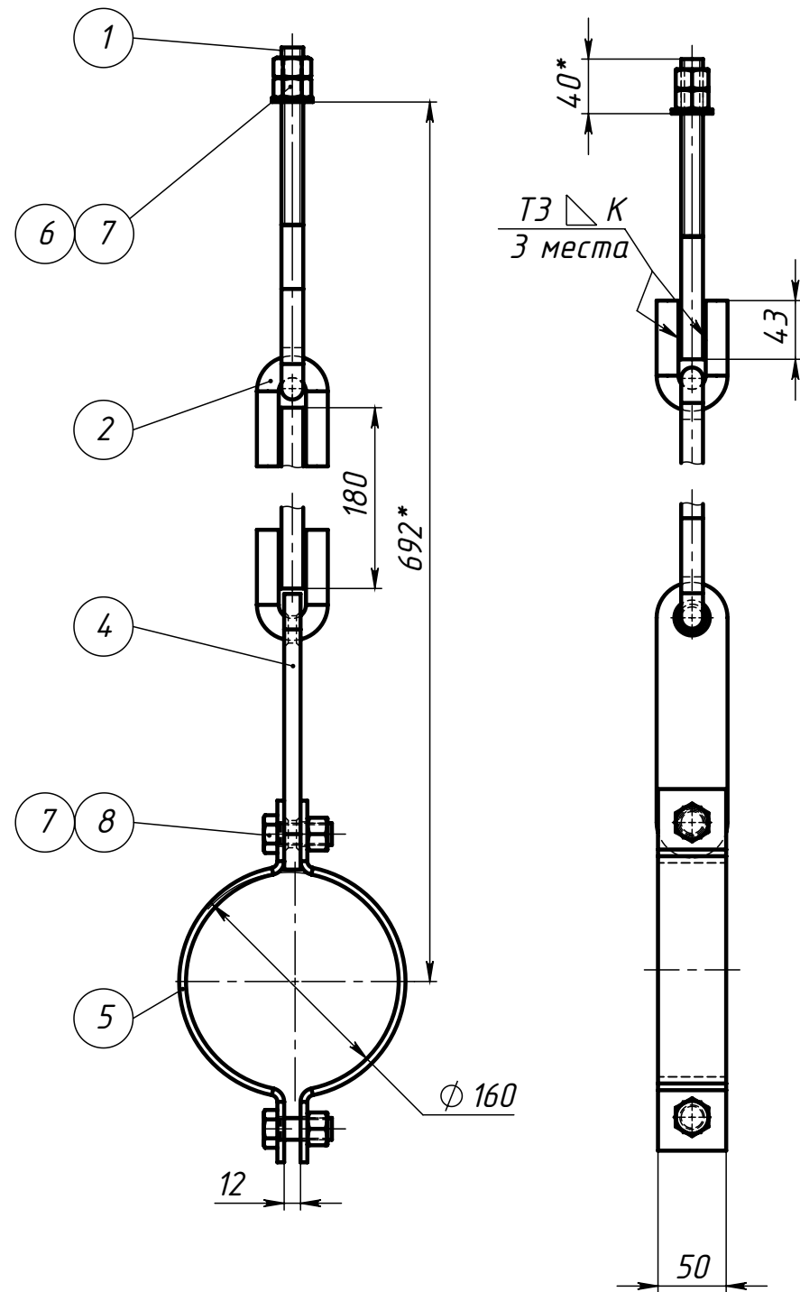
Поз.1 (Шпилька)
