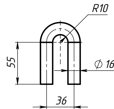
Поз.2 (Ушко 16)
