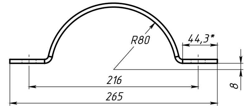
Поз.5 (Полухомут) развертка
