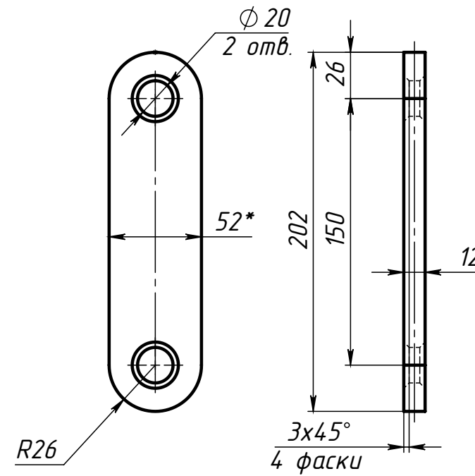
Поз.4 (Серьга 20)
